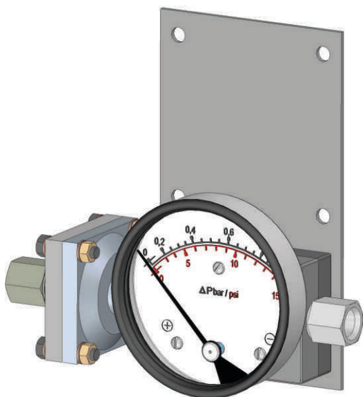
Aufbaumontage
