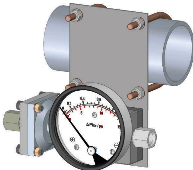
Horizontale Rohrmontage
