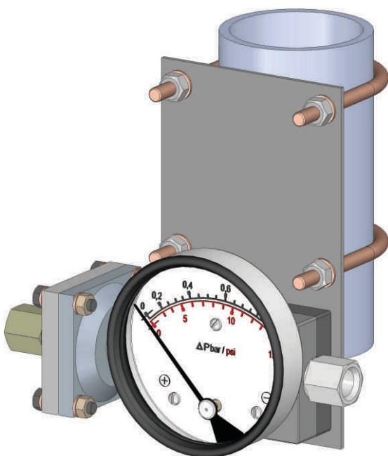
Vertikale Rohrmontage
