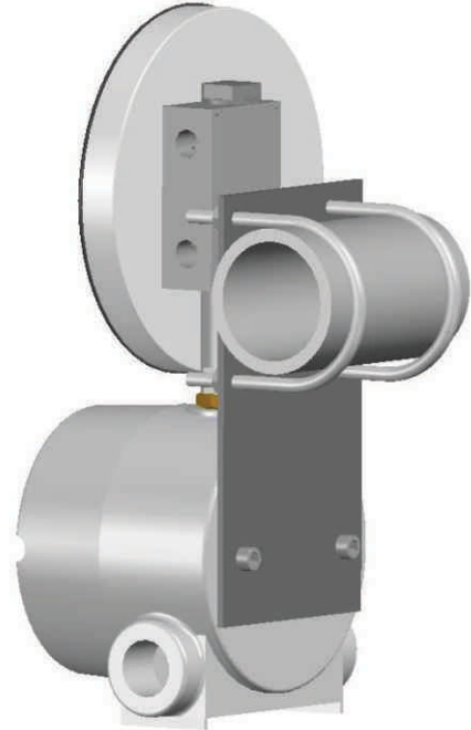
Horizontale Rohrmontage
